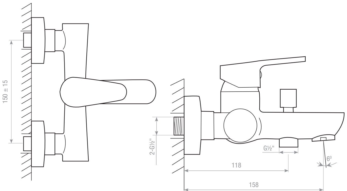
Desenho técnico (mm)
