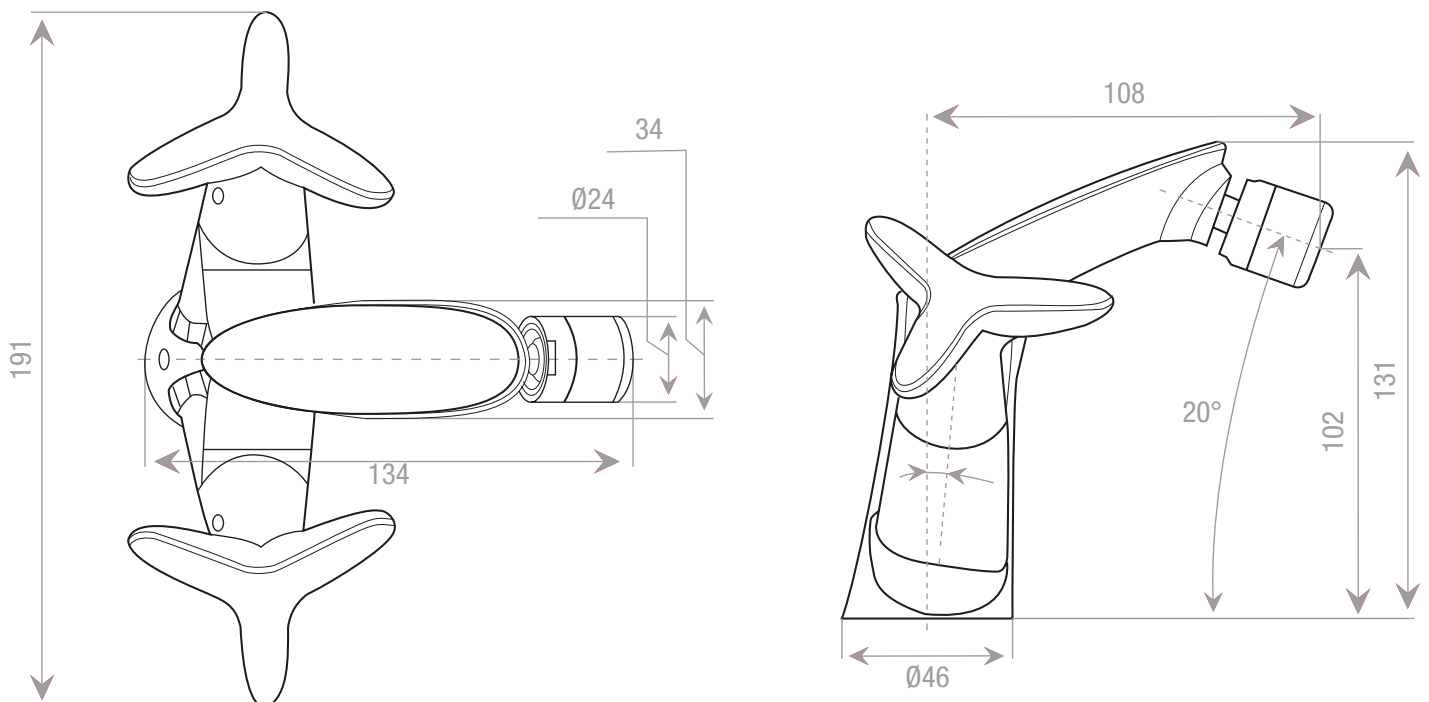
Desenho técnico (mm)
