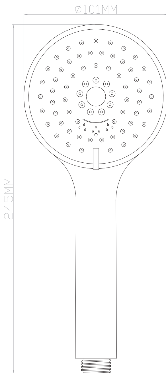
Desenho técnico
